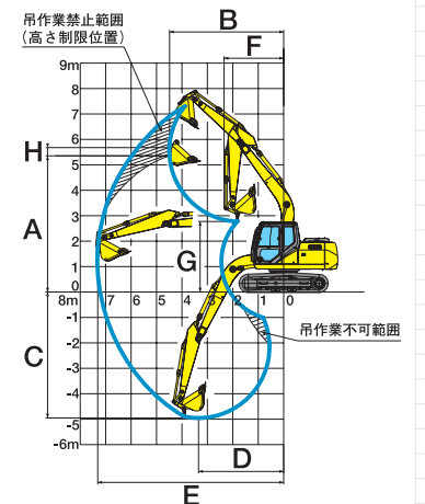
■作業範囲図
