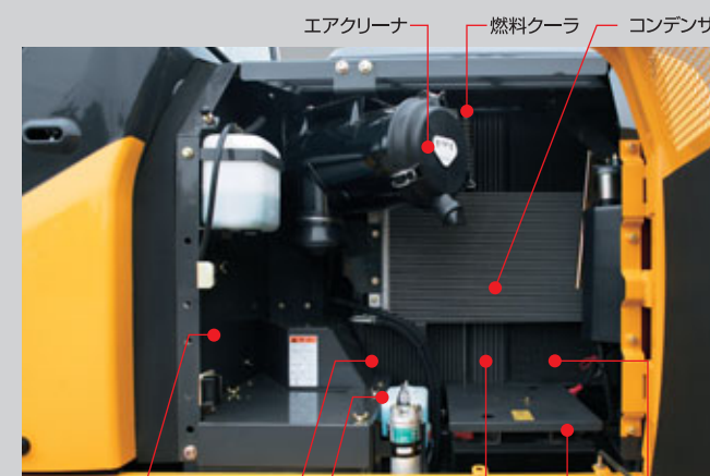
エアクリーナ 燃料クーラ コンデンサ エアコン外気フィルタ オイルクーラ ウォッシャータンク インタークーラ バッテリ ラジエータ
