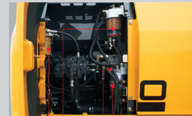
パイロットフィルタ オイルフィルタ 燃料フィルタ(ウォーターセパレータ付) 燃料プレフィルタ(ウォーターセパレータ付)
