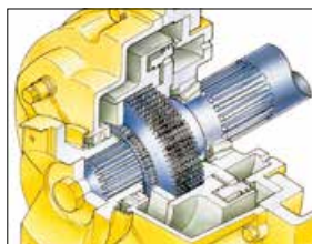
湿式ディスクパーキングブレーキ
