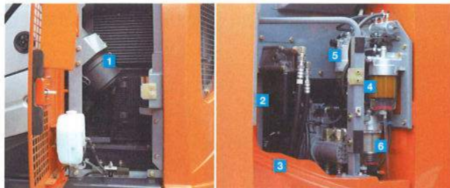
1 エアクリーナ 2 エンジンオイルフィルタ 3 パイロットフィルタ 4 燃料プレフィルタ 5 燃料メインフィルタ 6 ウォータセパレータ (オプション)
